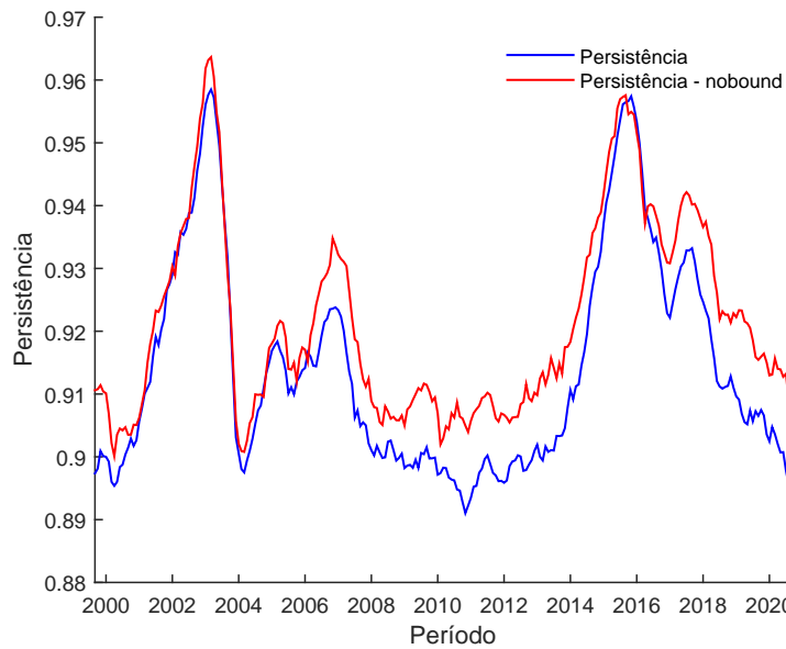
Figura 7 – Média a posteriori da persistência, \rho_t : modelo restrito (linha azul) e modelo irrestrito/nobound (linha vermelha).
