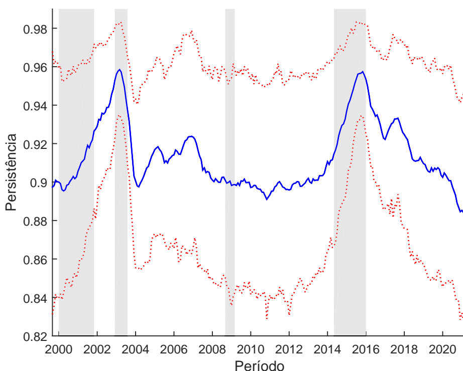
Figura 3 – Média a posteriori da persistência, \rho_t (linha azul); quantis 16 e 84% (linhas vermelhas); e cronologia mensal dos ciclos de negócios, segundo CODACE (áreas sombreadas).
