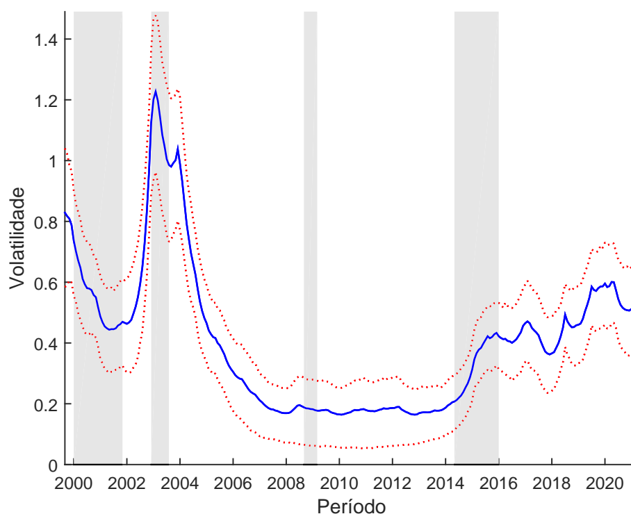
Figura 4 – Média a posteriori da volatilidade do gap da inflação (linha azul); quantis 16 e 84% (linhas vermelhas); e cronologia mensal dos ciclos de negócios, segundo CODACE (áreas sombreadas).
