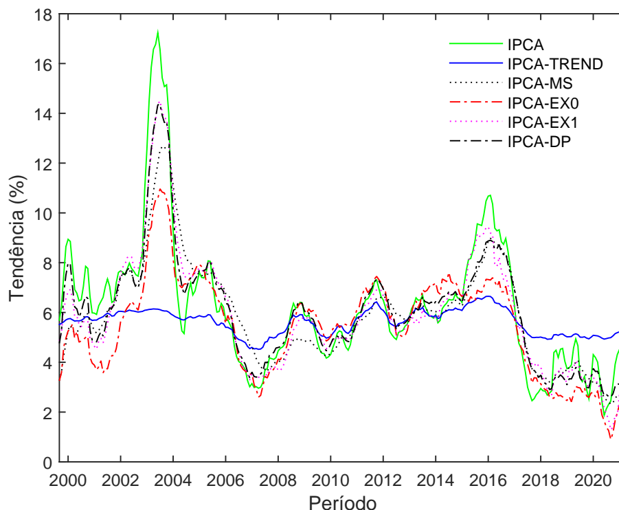
Figura 5 – Inflação (IPCA), tendência da inflação (IPCA-TREND), médias aparadas com suavização (IPCA-MS); por exclusão do subgrupo alimentação no domicílio e do segmento de administrados (IPCA-EX0); por exclusão de 10 dos 16 itens do subgrupo alimentação no domicílio, além dos itens combustíveis domésticos e combustíveis de veículos (IPCA-EX1); e dupla ponderação (IPCA-DP).
