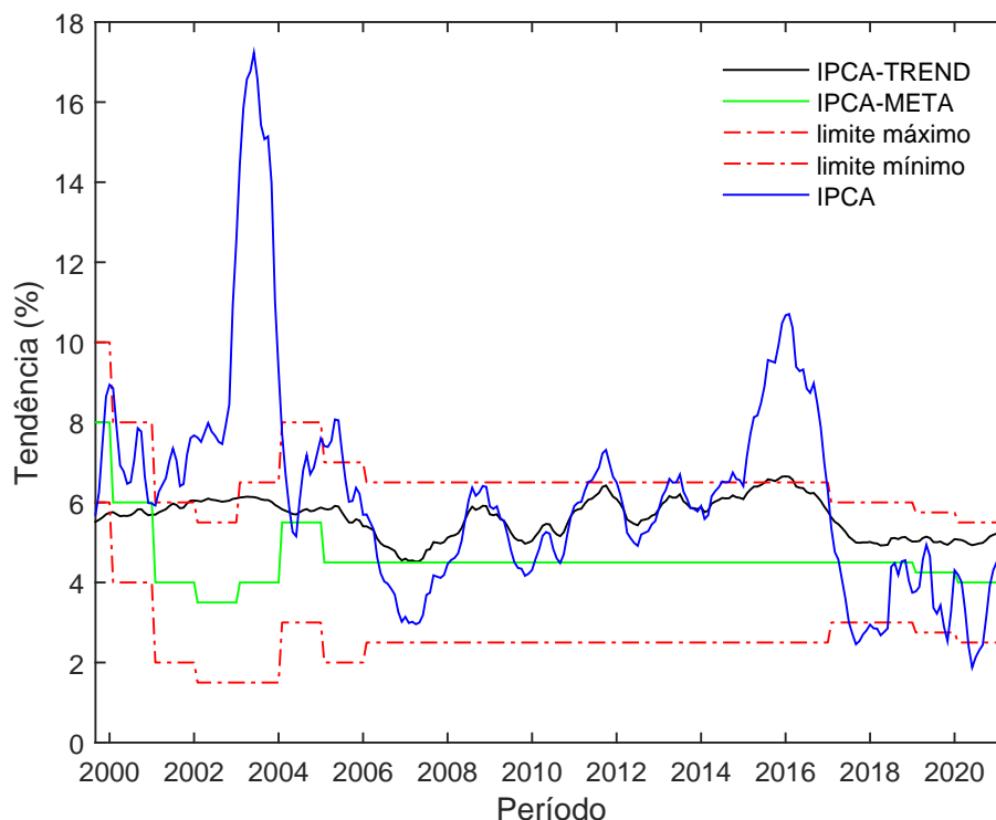
Figura 2 – Média a posteriori da tendência da inflação, \tau_t (IPCA-TREND); IPCA (em % 12 meses); Meta de inflação (IPCA-META); Limites do intervalo de tolerância da meta de inflação (máximo/mínimo).
