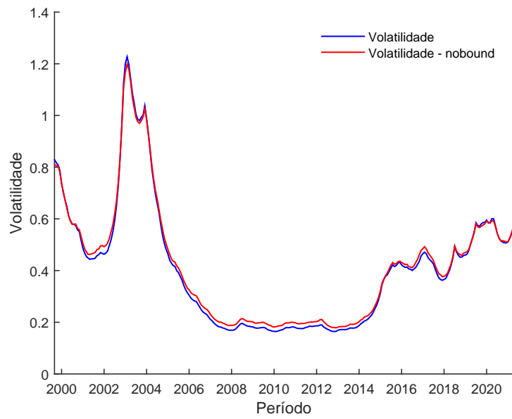
Figura 8 – Média a posteriori da volatilidade do gap da inflação: modelo restrito (linha azul) e modelo irrestrito/nobound (linha vermelha).
