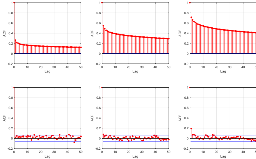
Figura 1 – Correlogramas das cadeias geradas para \tau_1 (esquerda), \tau_{107} (centro) e \tau_{213} (direita), antes (acima) e depois (abaixo) de serem espaçadas em lags de tamanho 1.000.
