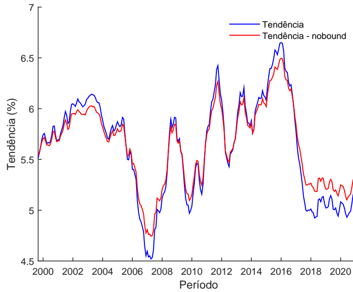
Figura 6 – Média a posteriori da tendência da inflação, \tau_t : modelo restrito (linha azul) e modelo irrestrito/nobound (linha vermelha).
